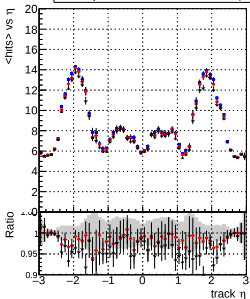
DQM_mkFit_baseline_lowPT DQM_mkFit_baseline6iter_lowPT DQM_mkFit_TT_RetrainV2_WP1_6iter_ep3_lowPT mean hits
