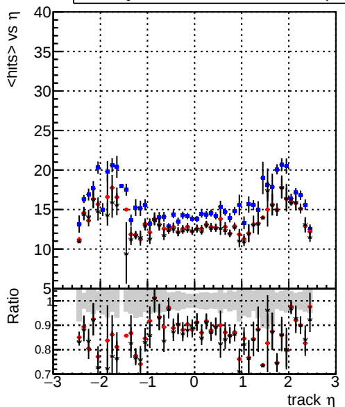
mean hits — DQM_mkFit_baseline_lowPT — DQM_mkFit_baseline_lowPT — DQM_mkFit_TT_RetrainV2_WP1_6iter_ep3_lowPT
