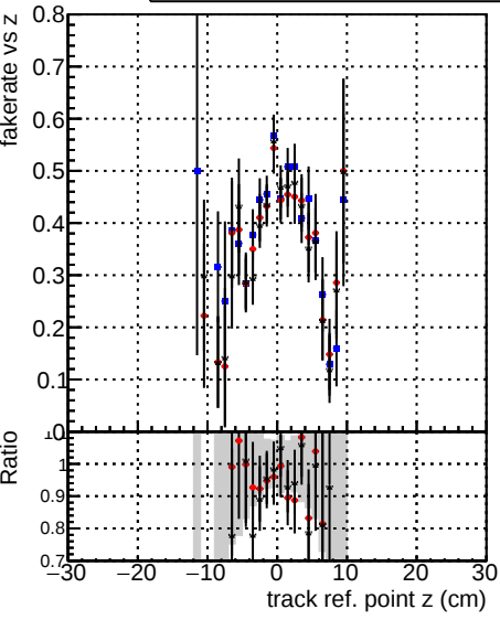
—●— DQM_mkFit_baseline_lowPT —●— DQM_mkFit_baseline6iter_lowPT —●— DQM_mkFit_TT_RetrainV2_WP1_6iter_ep3_lowPT
