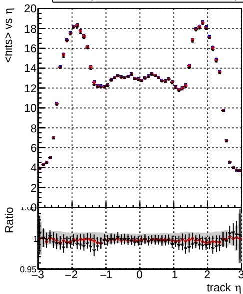
mean hit — DQM_mkFit_baseline_lowPT — DQM_mkFit_baseline6iter_lowPT — DQM_mkFit_TT_RetrainV2_WP1_6iter_ep3_lowPT
