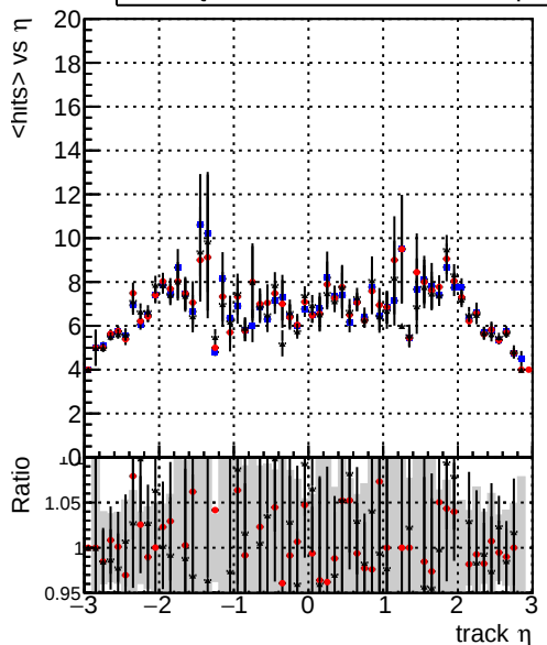
mean hit — DQM_mkFit_baseline_lowPT — DQM_mkFit_baseline6iter_lowPT — DQM_mkFit_TT_RetrainV2_WP1_6iter_ep3_lowPT
