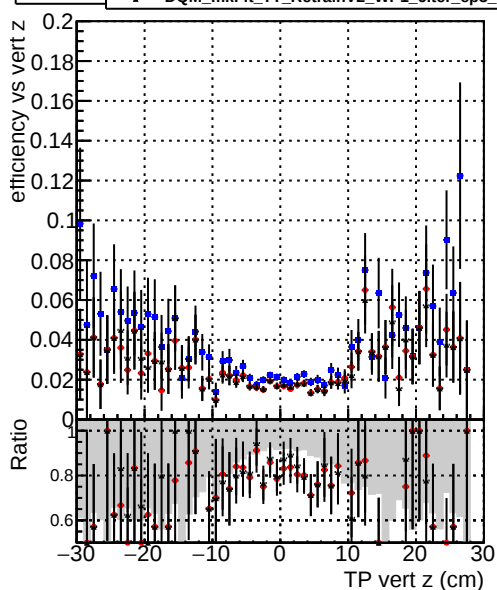
Efficiency vs. TP vert z — DQM_mkFit_baseline_lowPT — DQM_mkFit_baseline6iter_lowPT — DQM_mkFit_TT_RetrainV2_WP1_6iter_ep3_lowPT
