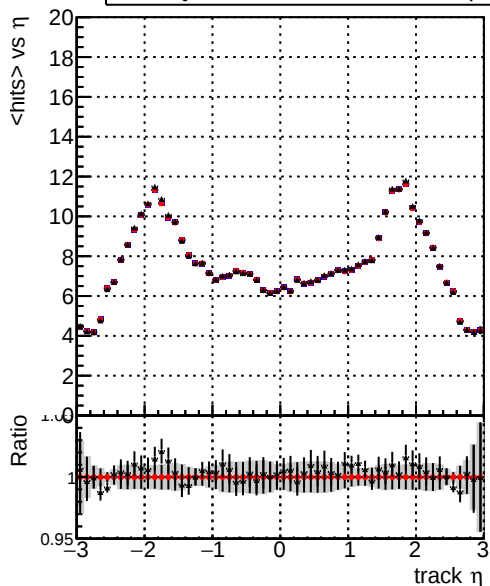
— DQM_mkFit_baseline_lowPT — DQM_mkFit_baseline6iter_lowPT — DQM_mkFit_TT_RetrainV2_WP1_6iter_ep3_lowPT
