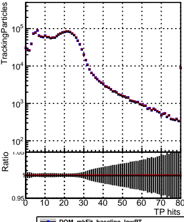
— DQM_mkFit_baseline_lowPT — DQM_mkFit_baseline6iter_lowPT — DQM_mkFit_TT_RetrainV2_WP1_6iter_ep3_lowPT
