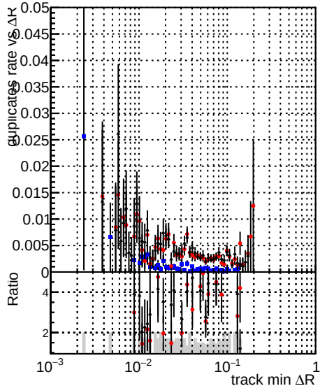
—●— DQM mkFit baseline_lowPT —●— DQM mkFit baseline6iter_lowPT —●— DQM mkFit TT_RetrainV2_WP1_6iter_ep3_lowPT
