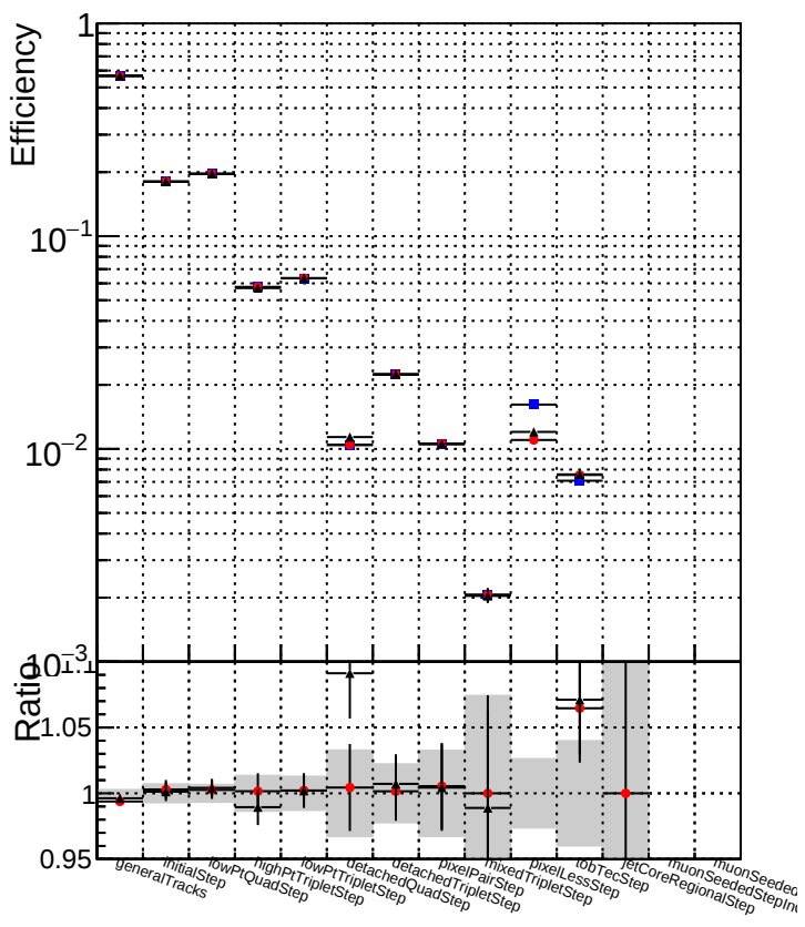
DQM_mkFit_baseline DQM_mkFit_baseline6iter DQM_mkFit_TT_RetrainV2_WP2_6iter_ep3
