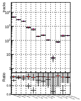
N of reco track vs. \chi^2 DQM mkFit baseline DQM mkFit baseline gitter DQM mkFit V2 WP2 6iter ep3
