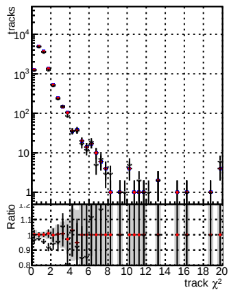
N of reco track vs. \chi^2 DQM mkFit baseline DQM mkFit baseline gitter DQM mkFit V2 WP2 6iter ep3
