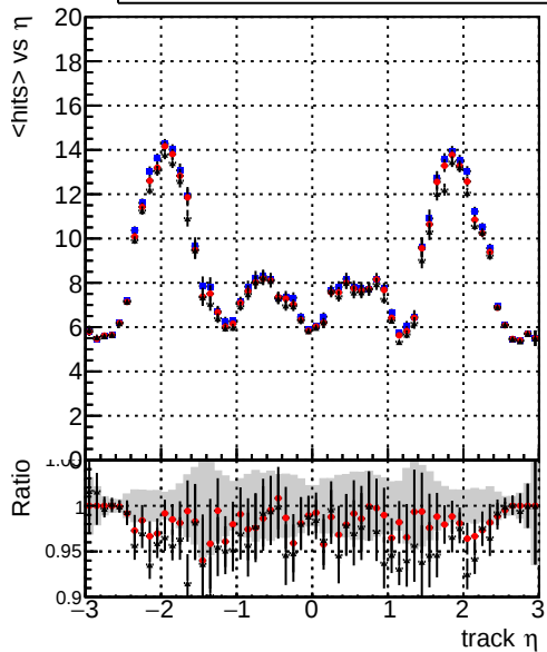
DQM_mkFit_baseline DQM_mkFit_baseline6iter DQM_mkFit_TT_RetrainV2_WP2_6iter_ep3 mean hit
