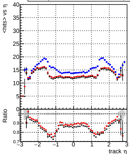
mean hit — DQM_mkFit_baseline — DQM_mkFit_baseline6iter — DQM_mkFit_TT_RetrainV2_WP2_6iter_ep3
