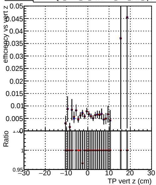
Efficiend —●— DQM_mkFit_baseline6iter —▲— DQM_mkFit_TT_RetrainV2_WP2_6iter_ep3
