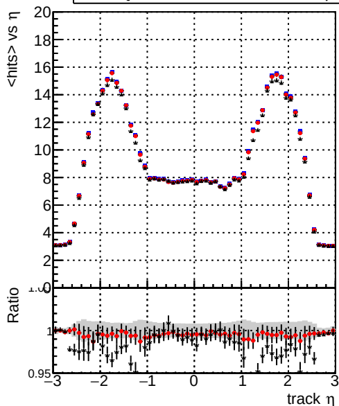
mean hits — DQM_mkFit_baseline — DQM_mkFit_baseline6iter — DQM_mkFit_TT_RetrainV2_WP2_6iter_ep3
