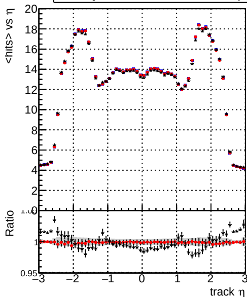
mean hit — DQM_mkFit_baseline — DQM_mkFit_baseline6iter — DQM_mkFit_TT_RetrainV2_WP2_6iter_ep3
