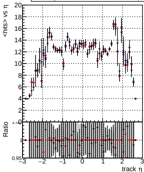
mean hits vs \eta — DQM_mkFit_baseline — DQM_mkFit_baseline6iter — DQM_mkFit_TT_RetrainV2_WP2_6iter_ep3
