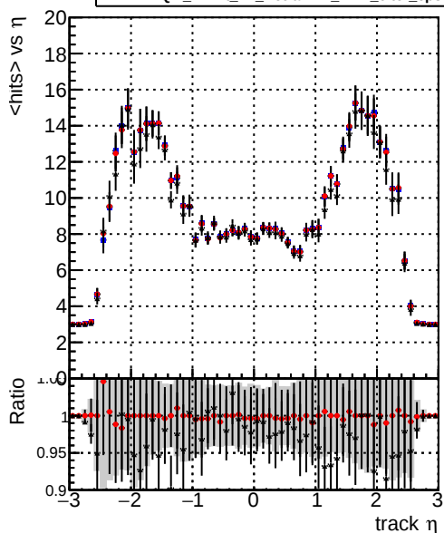
DQM_mkFit_baseline DQM_mkFit_baseline6iter DQM_mkFit_TT_RetrainV2_WP2_6iter_ep3
