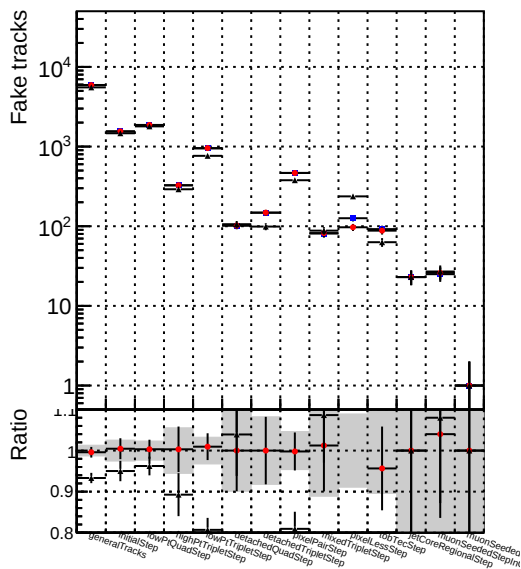
Number Model 1 DQM_mkFit_basellhe6iter 2 DQM_mkFit TT_RetrainV2_WP2_6iter_ep3
