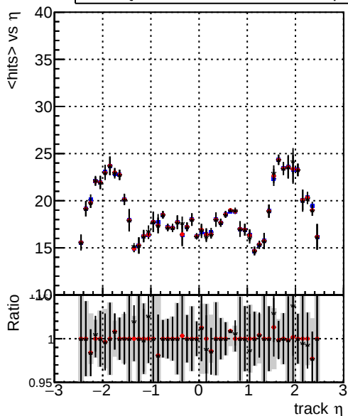
mean hit — DQM_mkFit_baseline — DQM_mkFit_baseline6iter — DQM_mkFit_TT_RetrainV2_WP2_6iter_ep3
