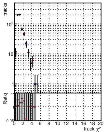
N of reco track vs. \chi^2 DQM mkFit baseline DQM mkFit baseline gitter DQM mkFit V2 Retrain V2 WP2 6iter ep3
