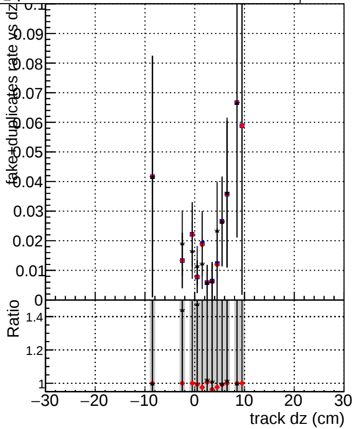
Legend: DQM_mkFit_baseline DQM_mkFit_baseline6iter DQM_mkFit_TT_RetrainV2_WP2_6iter_ep3
