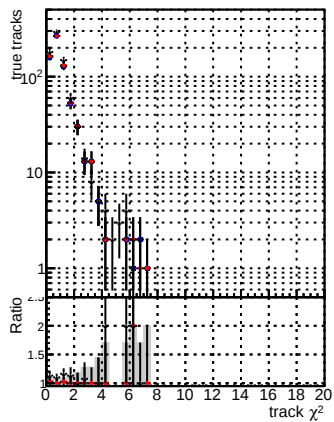
N of reco track vs. \chi^2 DQM mkFit baseline DQM mkFit baseline+gitter DQM mkFit V2 Retrain WP2 6iter ep3
