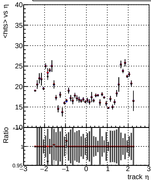
mean hits vs \eta DQM_mkFit_baseline DQM_mkFit_baseline6iter DQM_mkFit_TT_RetrainV2_WP2_6iter_ep3
