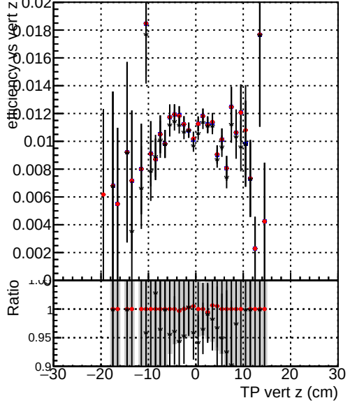
Efficiency vs. TP vert z (cm) — DQM_mkFit_baseline — DQM_mkFit_baseline6iter — DQM_mkFit_TT_RetrainV2_WP2_6iter_ep3
