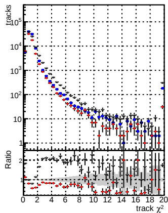
N of reco track vs. \chi^2 DQM mKF baseline DQM mKF 6iter DQM mKF 6iter ep3 WP2 6iter ep3
