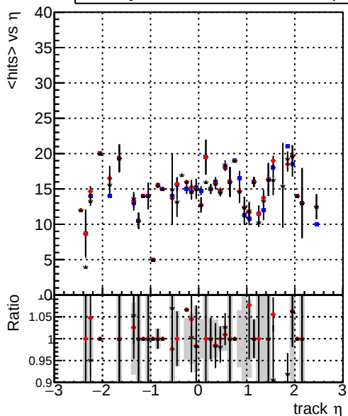
DQM_mkFit_baseline DQM_mkFit_baseline6iter DQM_mkFit_TT_RetrainV2_WP2_6iter_ep3
