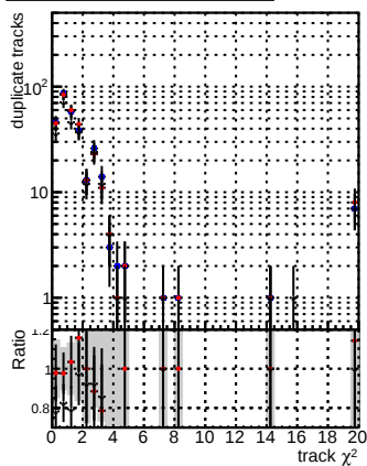
DOM mFit baseline DOM mFit baseline gitter DOM mFit WP2 6iter ep3 verSet
