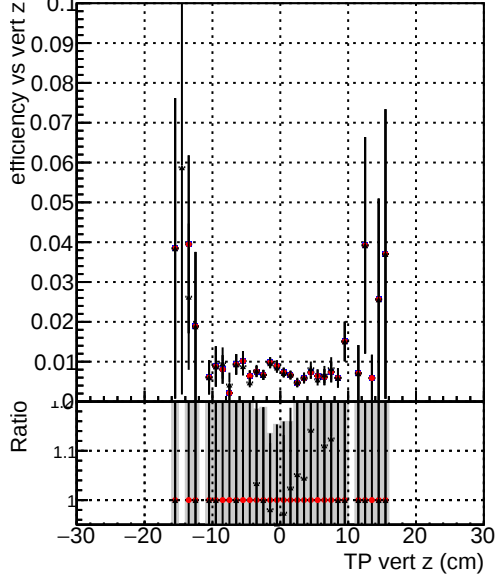
Efficiency vs vert z — DQM_mkFit_baseline — DQM_mkFit_baseline6iter — DQM_mkFit_TT_RetrainV2_WP2_6iter_ep3
