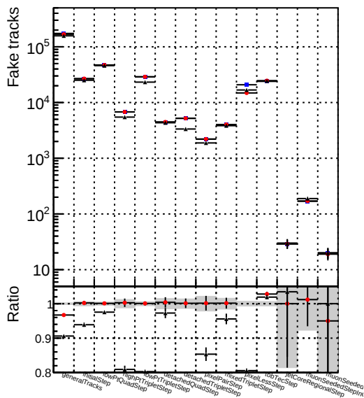
Number —●— DQM_mkFit_baseline6iter —▲— DQM_mkFit_TT_RetrainV2_WP1_6iter_ep3
