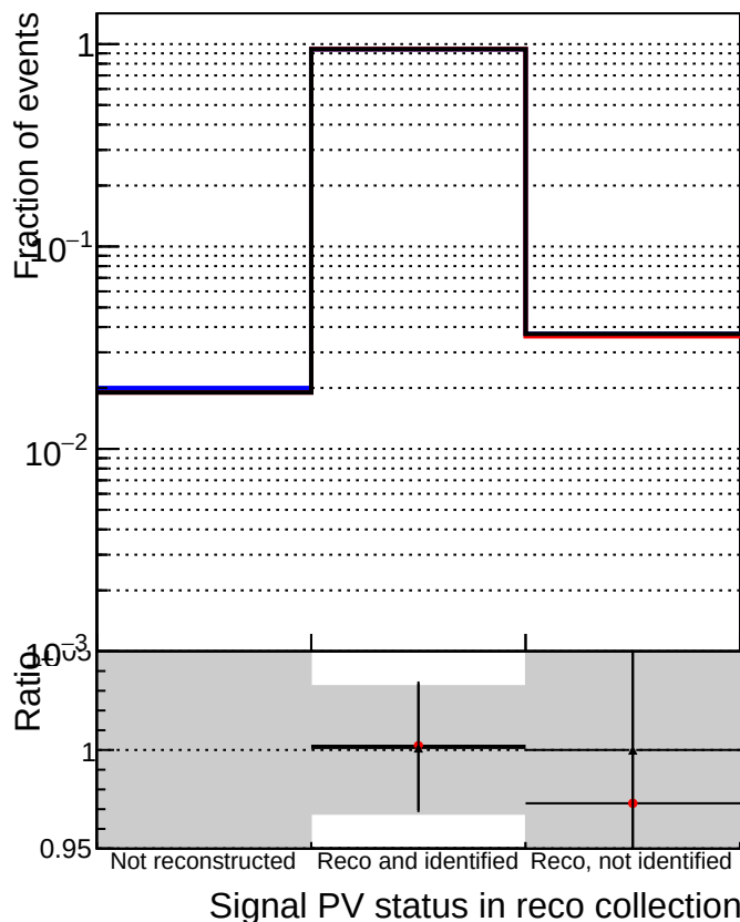
DQM_mkFit_baseline DQM_mkFit_baseline6iter DQM_mkFit_TT_RetrainV2_WP1_6iter_ep3
