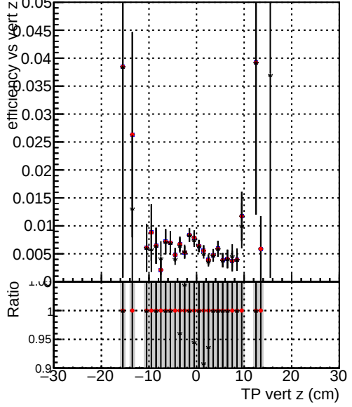
Efficiency vs vert z —●— DQM_mkFit_baseline —●— DQM_mkFit_baseline6iter —●— DQM_mkFit_TT_RetrainV2_WP1_6iter_ep3
