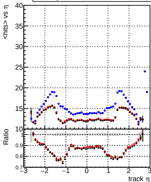
mean hits vs \eta — DQM_mkFit_baseline — DQM_mkFit_baseline6iter — DQM_mkFit_TT_RetrainV2_WP1_6iter_ep3
