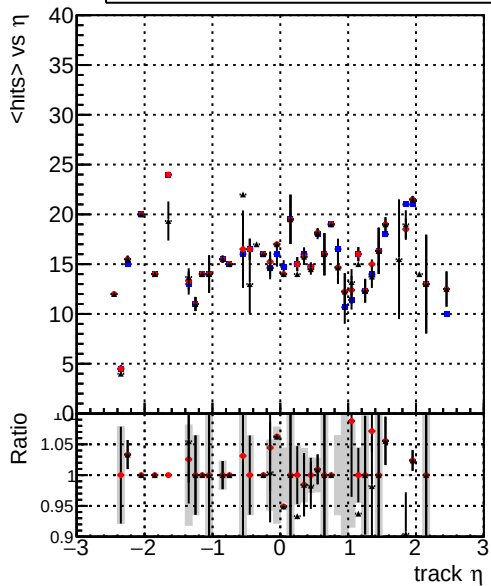
— DQM_mkFit_baseline — DQM_mkFit_baseline6iter — DQM_mkFit_TT_RetrainV2_WP1_6iter_ep3 mean hit
