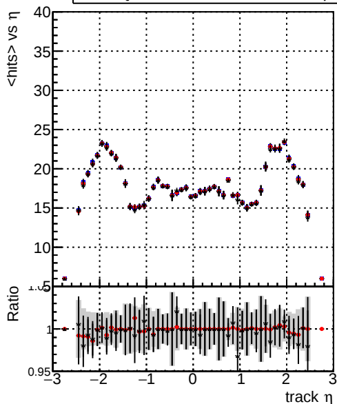
mean hit — DQM_mkFit_baseline — DQM_mkFit_baseline6iter — DQM_mkFit_TT_RetrainV2_WP1_6iter_ep3
