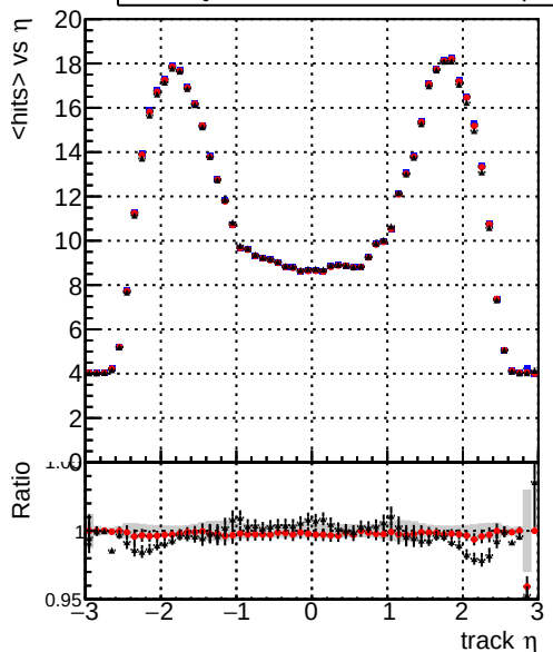
mean hits vs \eta — DQM_mkFit_baseline — DQM_mkFit_baseline6iter — DQM_mkFit_TT_RetrainV2_WP1_6iter_ep3
