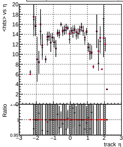
mean hits — DQM_mkFit_baseline — DQM_mkFit_baseline6iter — DQM_mkFit_TT_RetrainV2_WP1_6iter_ep3
