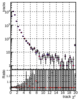
N of reco track vs. \chi^2 DQM mkFit baseline DQM mkFit baseline+gitter DQM mkFit V2 Retrain
