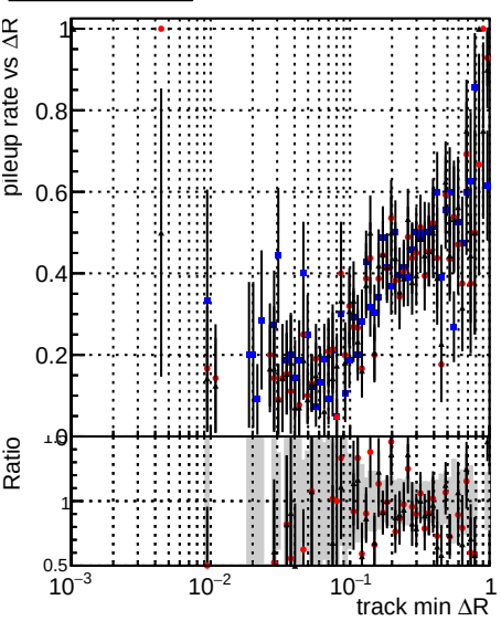
Legend: DQM mkFit baseline (blue dots), DQM mkFit baseline6iter (red dots), DQM mkFit TT_RetrainV2_WP1_6iter_ep3 (black dots)
