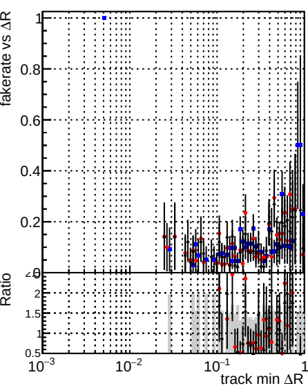
Legend: DQM mkFit baseline (blue dots), DQM mkFit baseline6iter (red dots), DQM mkFit TT_RetrainV2_WP1_6iter_ep3 (black dots)
