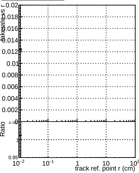
Fake rate vs verpos DQM_mkFit_baseline DQM_mkFit_baseline6iter DQM_mkFit_TT_RetrainV2_WP1_6iter_ep3
