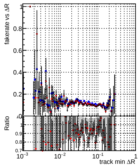
—●— DQM_mkFit_baseline —●— DQM_mkFit_baseline6iter —●— DQM_mkFit_TT_RetrainV2_WP1_6iter_ep3
