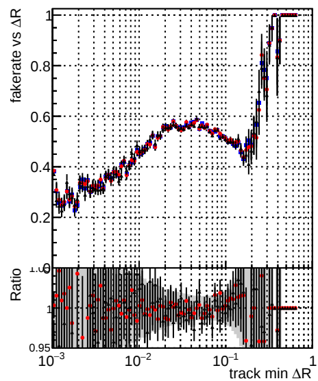
Legend: \blacksquare DQM_mkFit_baseline \bullet DQM_mkFit_baseline6iter \times DQM_mkFit_TT_RetrainV2_WP1_6iter_ep3
