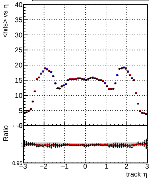
mean hits — DQM_mkFit_baseline — DQM_mkFit_baseline6iter — DQM_mkFit_TT_RetrainV2_WP1_6iter_ep3
