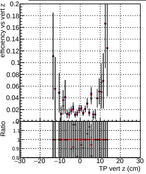
Efficiency vs TP vert z (cm) Legend: DQM_mkFit_baseline DQM_mkFit_baseline6iter DQM_mkFit_TT_RetrainV2_WP1_6iter_ep3
