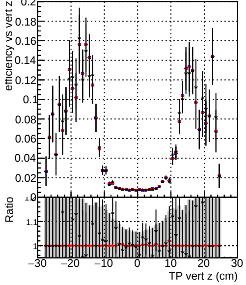
Efficiency vs. sim PV z — DQM_mkFit_baseline — DQM_mkFit_baseline6iter — DQM_mkFit_TT_RetrainV2_WP1_6iter_ep3
