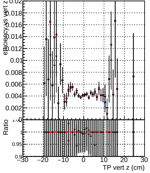
Efficiency vs TP vert z — DQM_mkFit_baseline — DQM_mkFit_baseline6iter — DQM_mkFit_TT_RetrainV2_WP1_6iter_ep3
