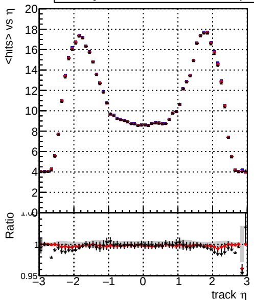
mean hit — DQM_mkFit_baseline — DQM_mkFit_baseline6iter — DQM_mkFit_TT_RetrainV2_WP1_6iter_ep3
