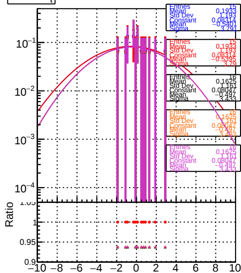
DOM mkFit5 XiMinus NORU base trainOldFiles125 v2 prelimWPM epoch4 trainOldFiles125 v2 prelimWPM epoch4
