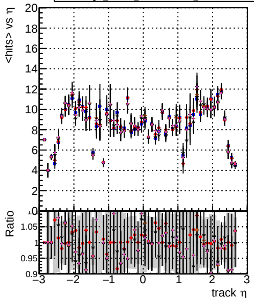
mean hits DQM mkFit5 X iMinusNOPU_base DQM mkFit5 X iMinusNOPU_retrainOldFiles125_v2_prelimWPM_epoch4 DQM mkFit5 X iMinusNOPU_base DQM mkFit6 X iMinusNOPU_retrainOldFiles125_v2_prelimWPM_epoch4 DQM mkFit5 X iMinusNOPU_retrainOldFiles125_v2_ANDLessRetrain_epoch4
