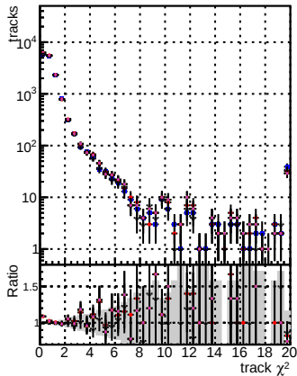
N of reco track vs. s TrainOldFiles125 v2 prelimWPM epoch4 TrainOldFiles125 v2 prelimWPM epoch4 TrainOldFiles125 v2 ANDLessReco epoch4
